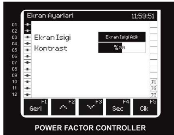
Şekil 10: Ekran Ayarları Menüsü
