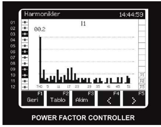
Şekil 22: Harmonikler
