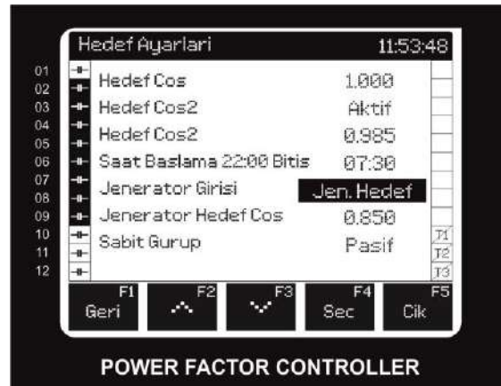
Şekil 7: Hedef Ayarları Menüsü
