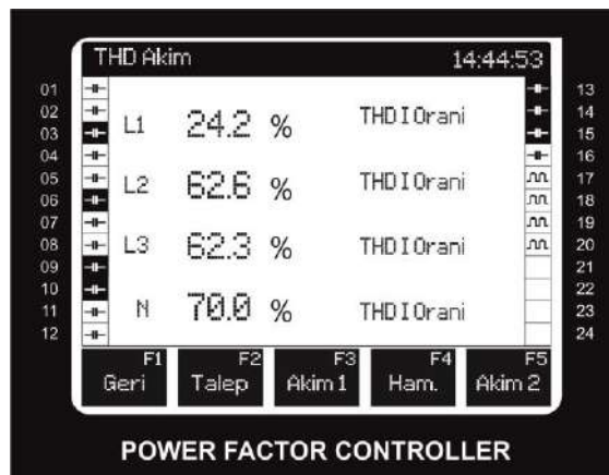
Şekil 21: THD Akım
