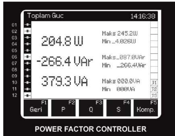
Şekil 14: Toplam Güç Ekranı
