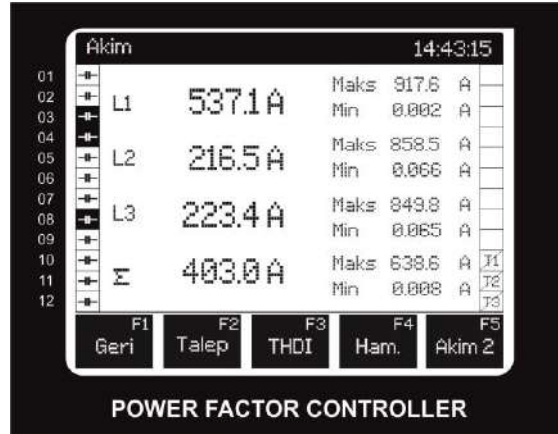
Şekil 19: Akım Ekranı
