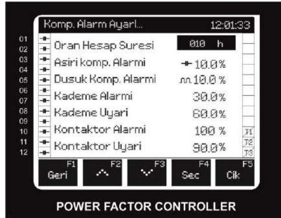
Şekil 8: Komp. Alarm Ayarları Menüsü
