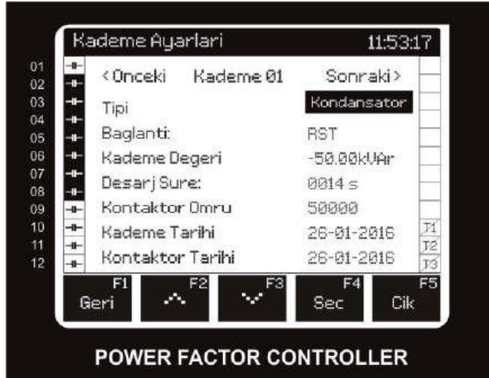
Şekil 5: Kompanzasyon Ayar Ekranı- Parametre Başlıkları
