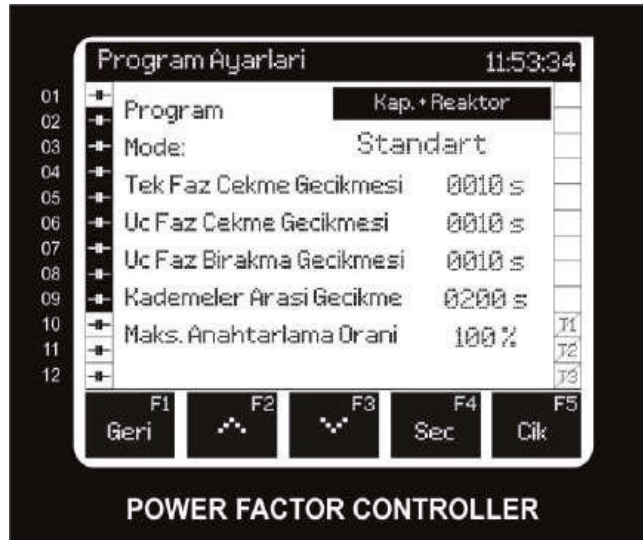
Şekil 6: Program Ayarları Menüsü
