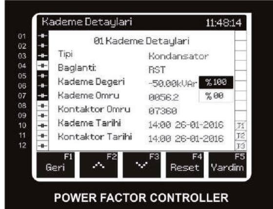
Şekil 12: Kademe Detayları Menüsü
